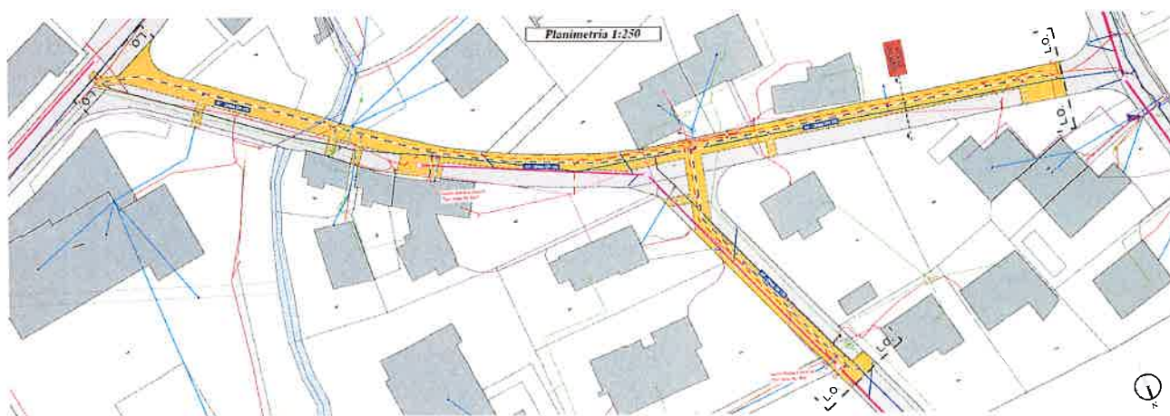
Progetto: condotte e pavimentazione
